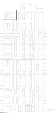
Fasade øst
